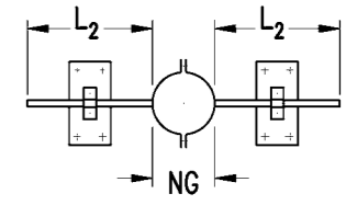
21 Rohrdachstütze HAL 9.11.33
