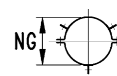
20 3-Punkt-Abspannung HAL 9.11.53
