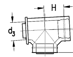
20 Winkelstück 87° Prüfföpfung waagrecht WPU 2.22.87
