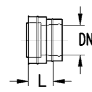
17 Reduzierstück USU 4.19.03
