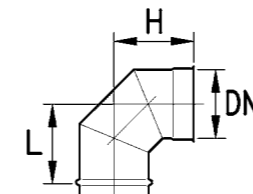
38 Bogen 90° / 87° BSK / BSS 2.11.90 / 87
