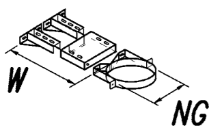
7 Wandhalter W = 210 - 263 mm
