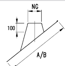
18 Führungsstutzen 28° - 50° FGS 6.30.16
