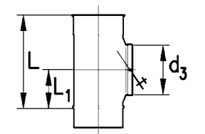
39 Nebenlufteinrichtung* NEK / NES 7.42.03
