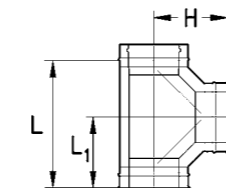
9 Einlaßstück 90° ATU 3.13.90
