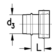
16 Übergang 1 auf 3-schalig / Kesselanschluss USU 5.16.13
