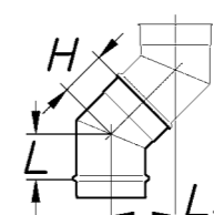
38 Bogen 45° / 30° / 15° BSK / BSS 2.11.45 / 30 / 15
