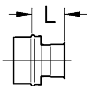
30 Reduzierung USK/USS 4.19.03
