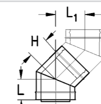
22 Bogen 45° / 30° / 15° BSU 2.11.45 / 30 / 15
