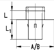
3 Abdeckung* mit Dehnungsausgleich AKU 6.50.23
