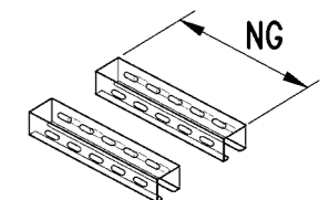
15 Trägerprofil HAL 9.15.51 - 54
