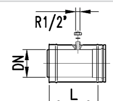
24 Abgasrohr mit Meßnippel ROU 1.18.13
