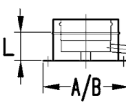
10 Kondensatschale KOU 6.31.13
