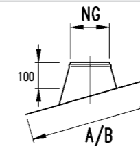
17 Führungsstutzen 5° - 27° FGS 6.30.15
