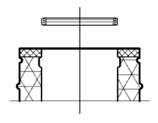
15 Dichtung montiert DIM 5.24.78
