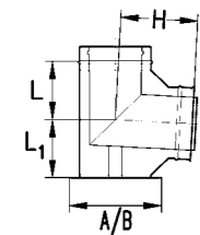
7 Einlaßstück 87° ESU 2.40.87
