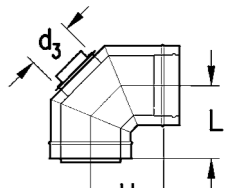
21 Bogen 90° * mit Prüfföpfung BPU 2.30.90
