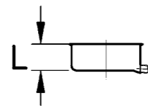
31 Kondensatschale KOK / KOS 6.31.13
