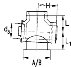
8 Einlaßstück 87° mit Prüfföpfung ESU 2.41.87
