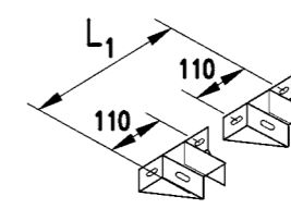
14 Fuß 80 HAL 9.15.42
