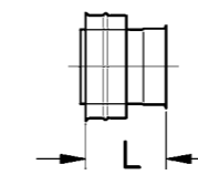
19 Übergangstück 3-schalig auf 1-schalig USU 5.16.23
