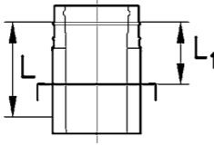
5 Stützrohr mit Ausgleichstutzen* SZU 9.21.13
