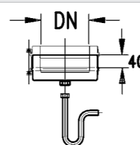
11 Rußtopf ohne Siphon* VDU 6.32.03
