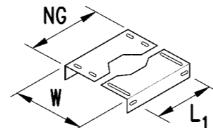
9 Unterfütterung W = bis 200 mm HAL 9.15.23
